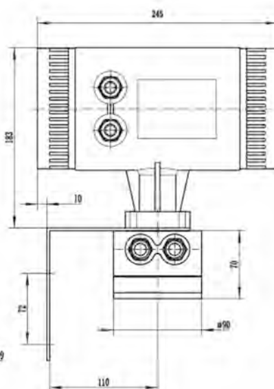
Раздельный преобразователь
