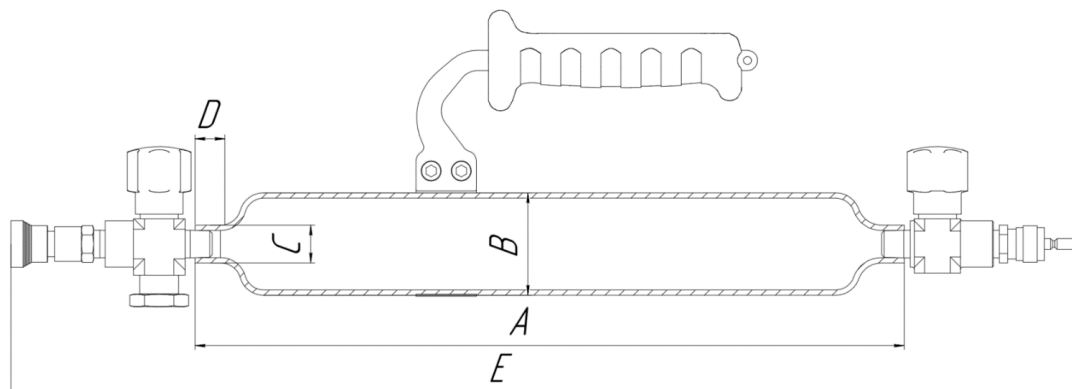
Рис. 1. Размеры цилиндра, необходимые для подбора Кейса.
