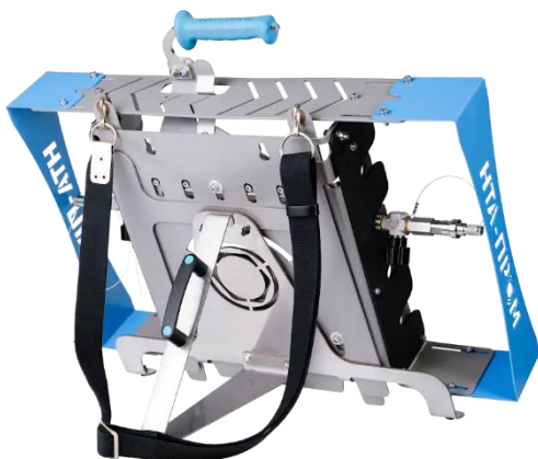
Рис. 5. Плечевой ремень.
