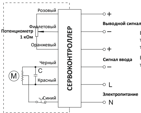
ТИП G: Цепь управления постоянного тока (с переключателем пассивного контакта)
