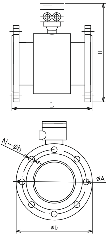
Чертеж раздельного электромагнитного расходомера DN15–DN600 с фланцем стандарта DIN
