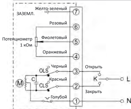
ТИП E: С сервоконтроллером
